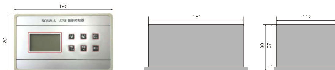
NQ6W外形及安装尺寸
