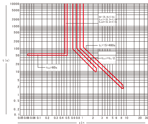
图3 负荷监测及控制(1个负荷限制和1个负荷重合的保护特性)
