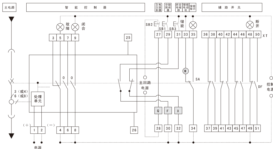
CFW3-2500~6300辅助开关由四常开四常闭独立触头组成的二次回路接线图
