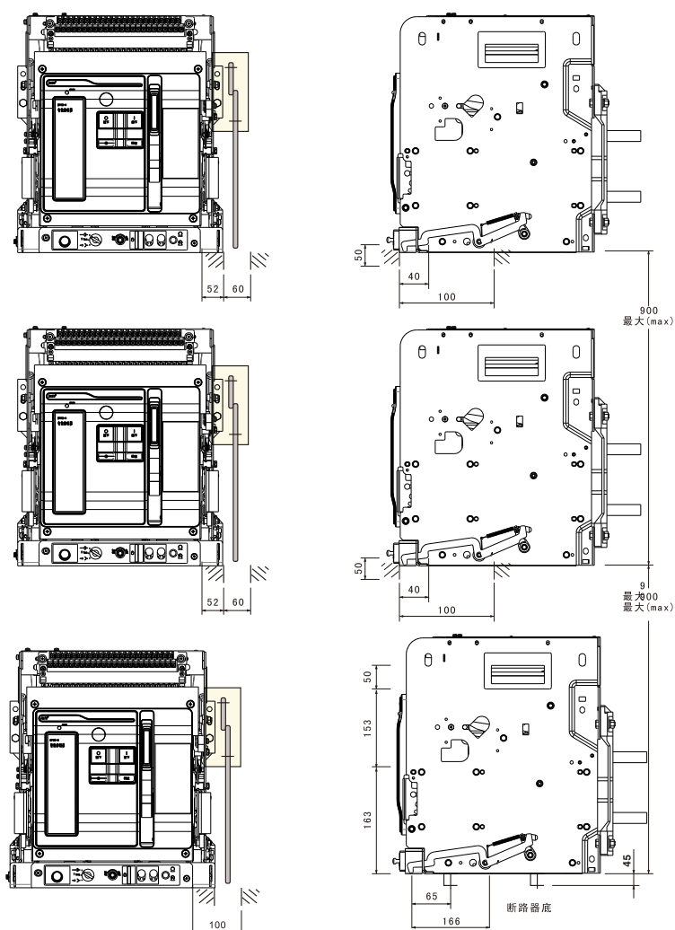
图7、叠装断路器联锁(图7为用联杆联锁的3个叠装断路器。如2个断路器联锁只需去除最上面的断路器。)
