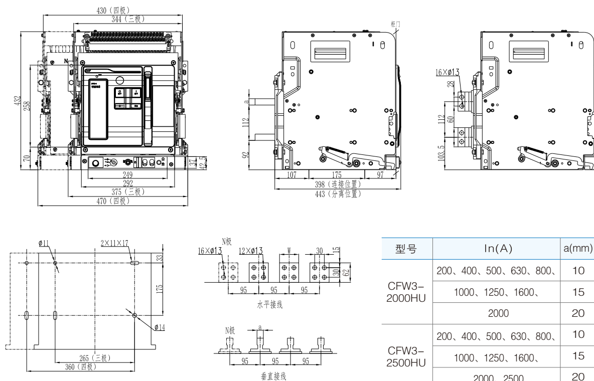
抽屉式断路器安装尺寸及外形尺寸(CFW3-2000HU、2000HU/4、CFW3-2500HU、2500HU/4)
