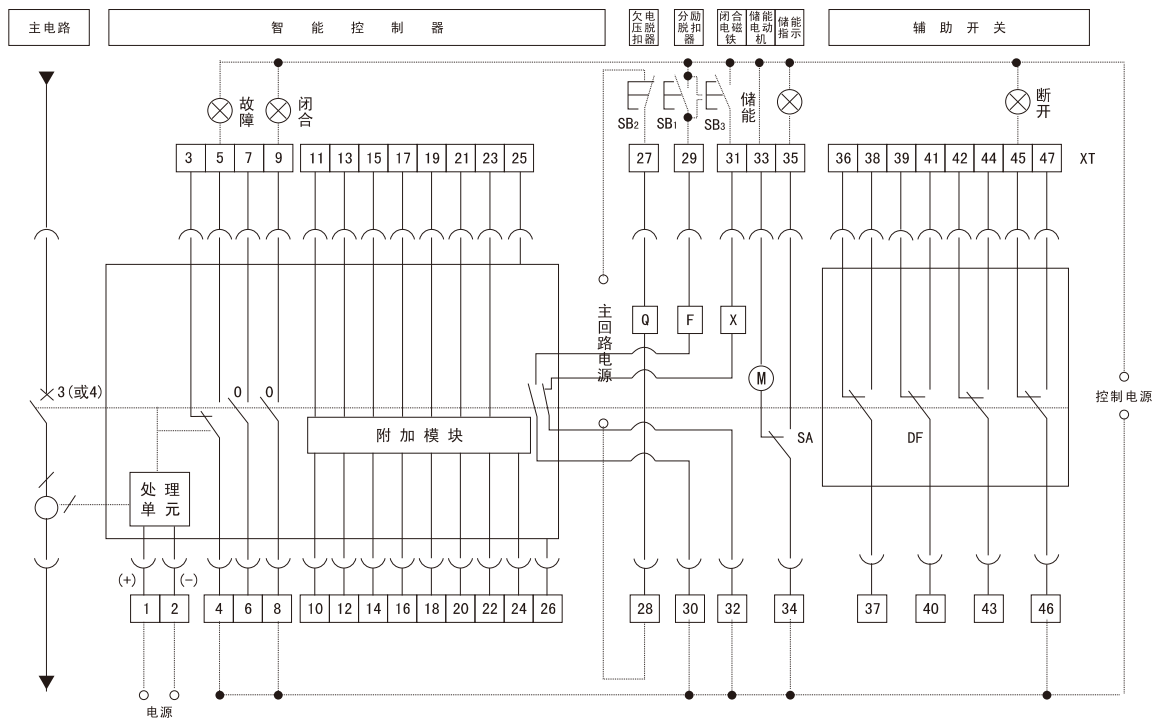
CFW3-2500HU~6300HU控制器为M型带通讯功能线路图
