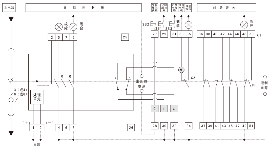
CFW3-2500HU~6300HU辅助开关由四常开四常闭独立触头组成的二次回路接线图
