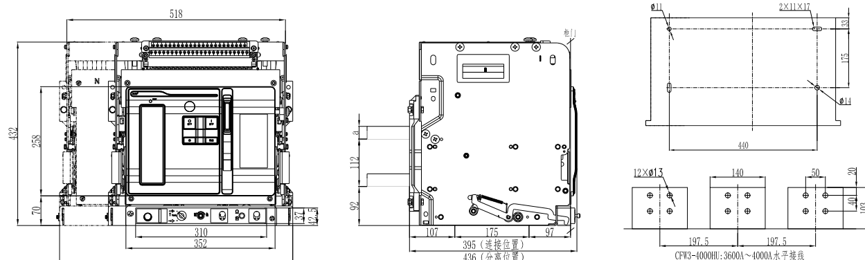
抽屉式断路器安装尺寸及外形尺寸(CFW3-4000HU: 3600A~4000A)
