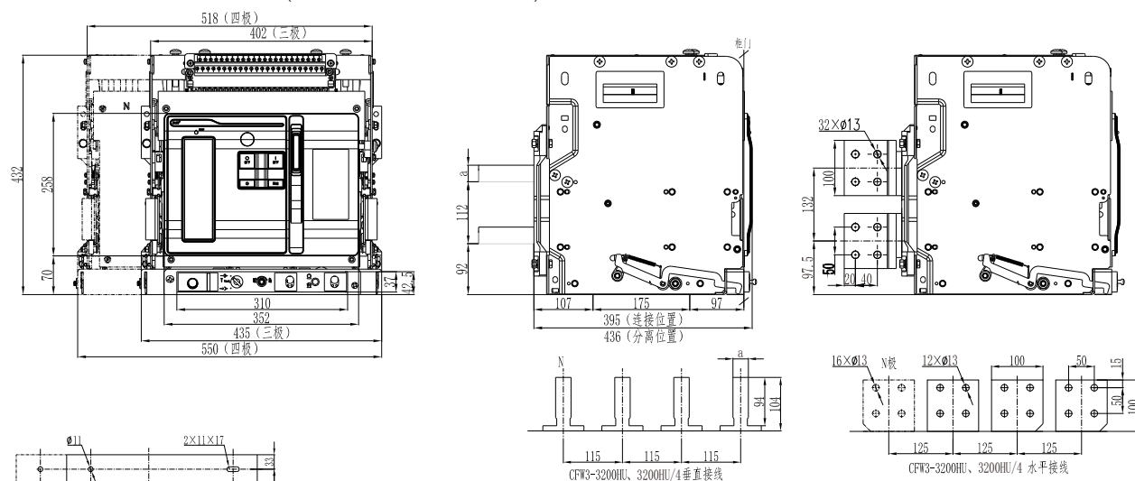
抽屉式断路器安装尺寸及外形尺寸(CFW3-3200HU、3200HU/4)
