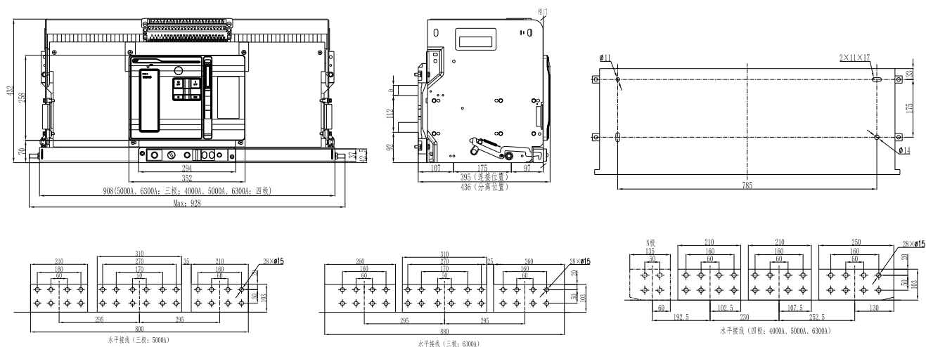
抽屉式断路器安装尺寸及外形尺寸(CFW3-6300HU、6300HU/4)
