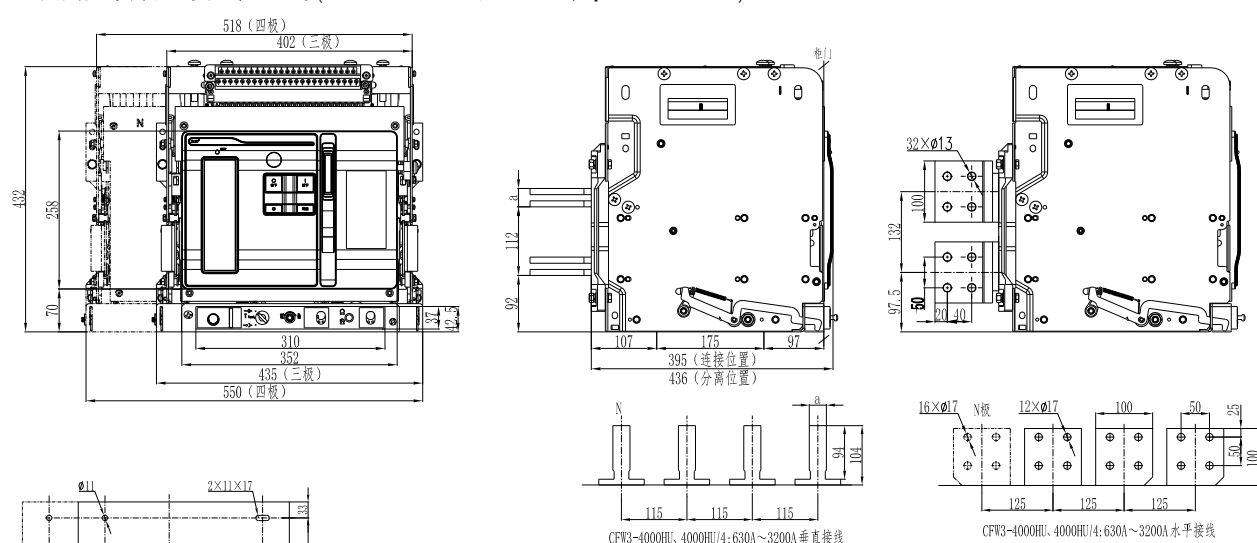
抽屉式断路器安装尺寸及外形尺寸(CFW3-4000HU、4000HU/4: 630A~3200A)
