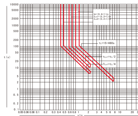
图4 负载监测及控制(双负荷限制的保护特性)
