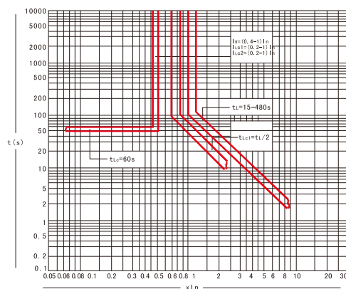
图3 负载监测及控制(1个负荷限制和1个负荷重合的保护特性)
