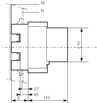
• CFM5-100~630 3P
