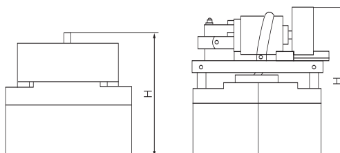
图5 装电动操作机构后的外形尺寸
