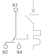
报警开关SD
