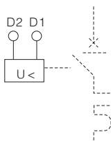
过欠压脱扣器MV+MN
