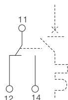
辅助开关OF
