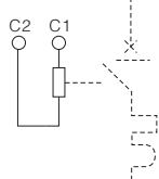
分励脱扣器+辅助开关
