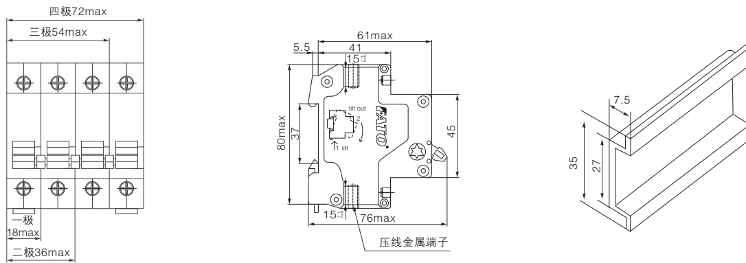
图1 CFH2-125小型隔离开关外形及安装尺寸
