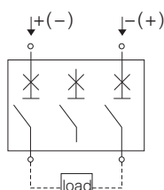
图2 3P外形(可选B1接线)
