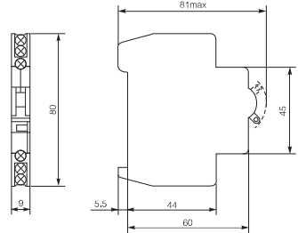
CFB3-FB辅助报警触头
