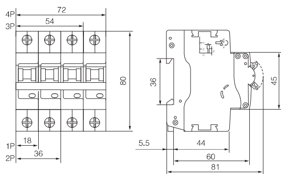
• CFB3-63小型断路器
