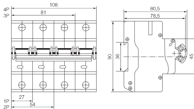
• CFB3-125小型断路器
