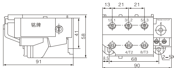
图3 JR36B-63
