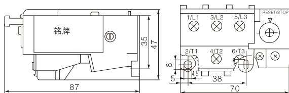
图2 JR36B-20、32
