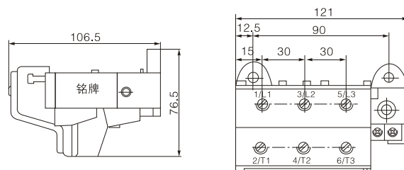
图4 JR36B-160
