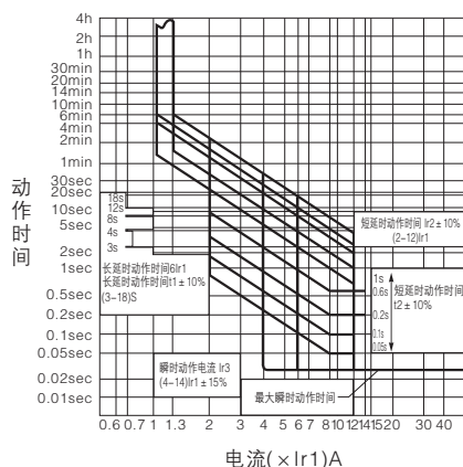
电子式过流短路保护特性曲线
