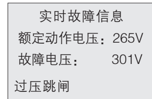
图10 过压跳闸界面： 过压跳闸：当前电压大于档位设定的电压时，显示过压故障。
