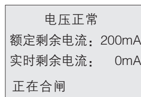
图2 合闸显示界面： 按“合闸”键断路器开始合闸
