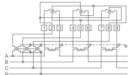
DX862/DX864型经电压、电流互感器接入式
