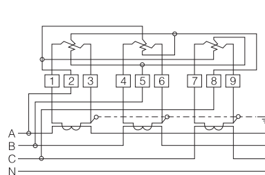
DX862/DX864型经万用电流互感器接入式
